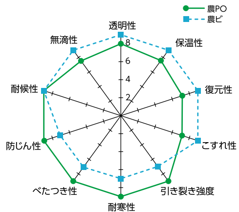
図2 農ビと農POの性能比較
