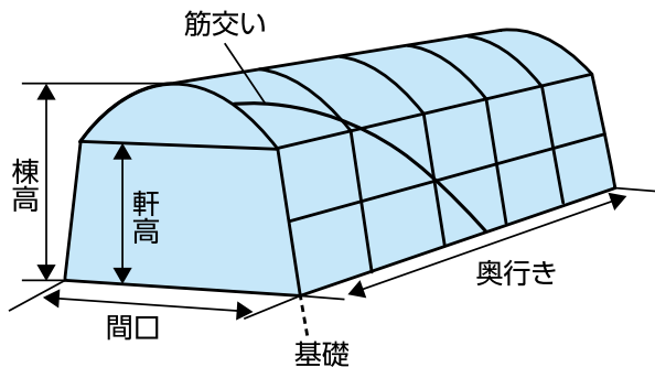
図1 ハウスの構造
